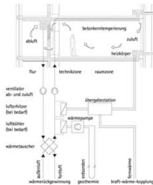
Energiekonzept/Anlagenschema
